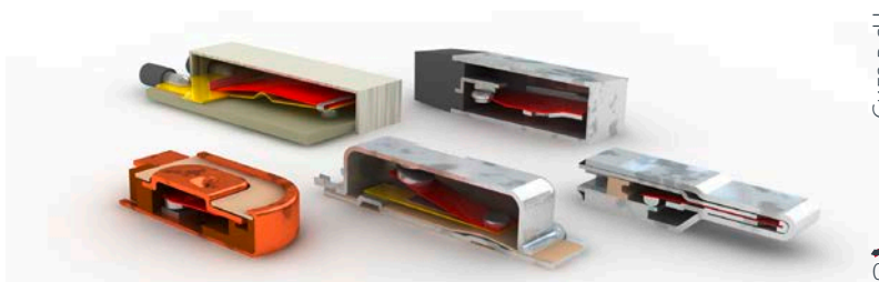
Рис. 1: Примеры систем размыкающихся термоограничителей, автоматически возвращающихся в исходное положение и чувствительных по току: простые язычковые выключатели без дополнительной пружинной шайбы
