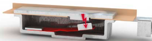
Рис. 3: Термоограничитель без дополнительной пружинной шайбы. В результате этого пережимаются контактирование и опасность возникновения световой дуги.
